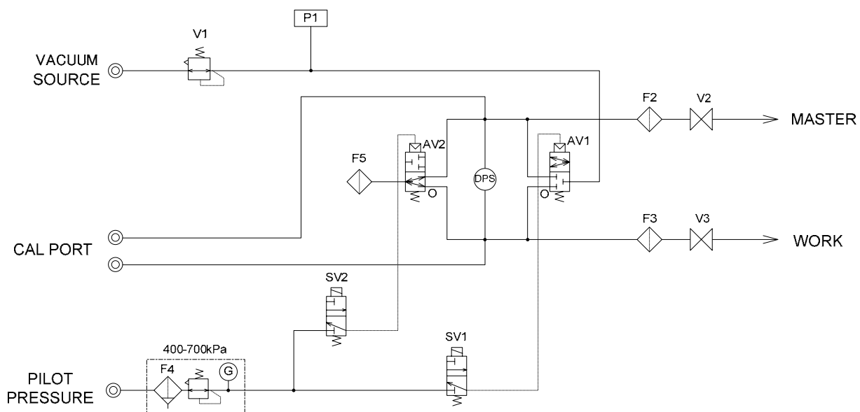
(b) 空氣回路圖 負壓用(V)
