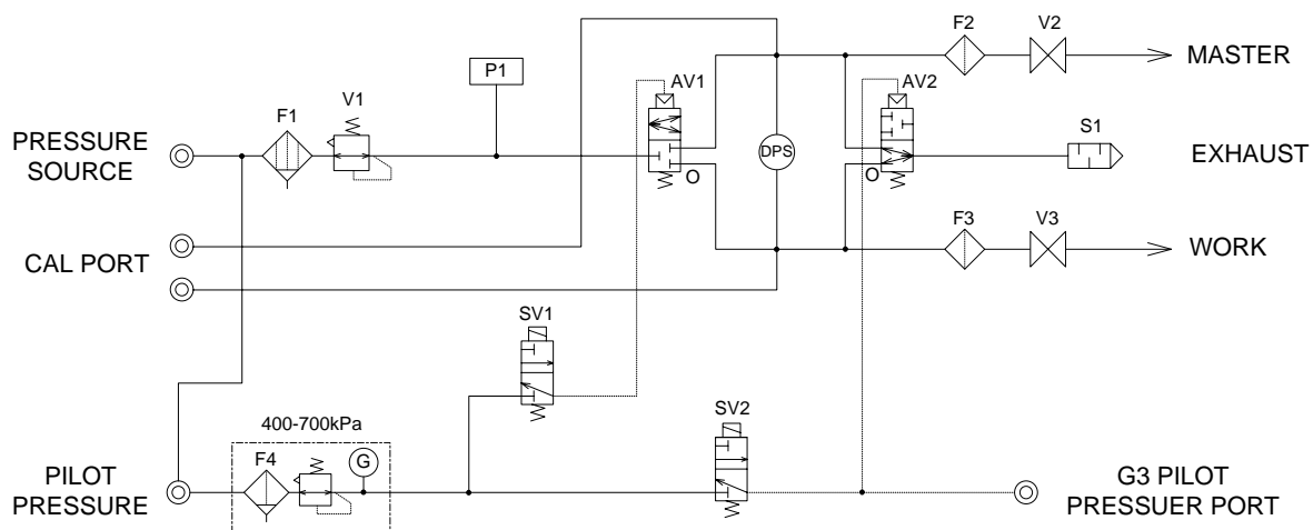
(a) 空氣回路圖 低壓用(L)、中壓用(M)
