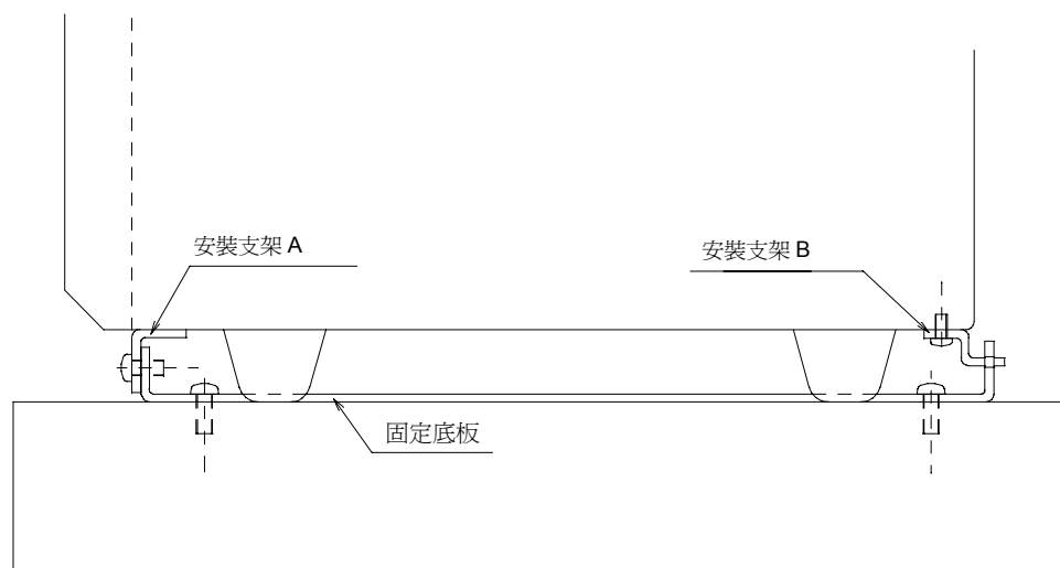
安裝金屬支架
