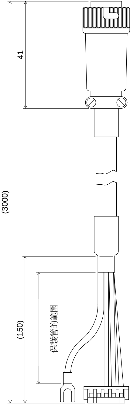
1.標準連接線外觀圖
